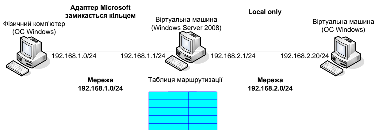
Рис. 2 – Схема мережі з маршрутизатором
