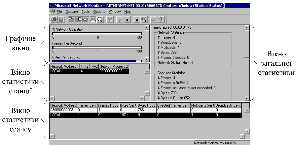
Рис. 3 – Елементи вікна Network Monitor
