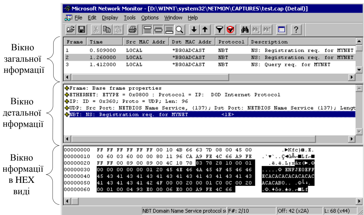
Рис. 4 – Елементи вікна Summary
